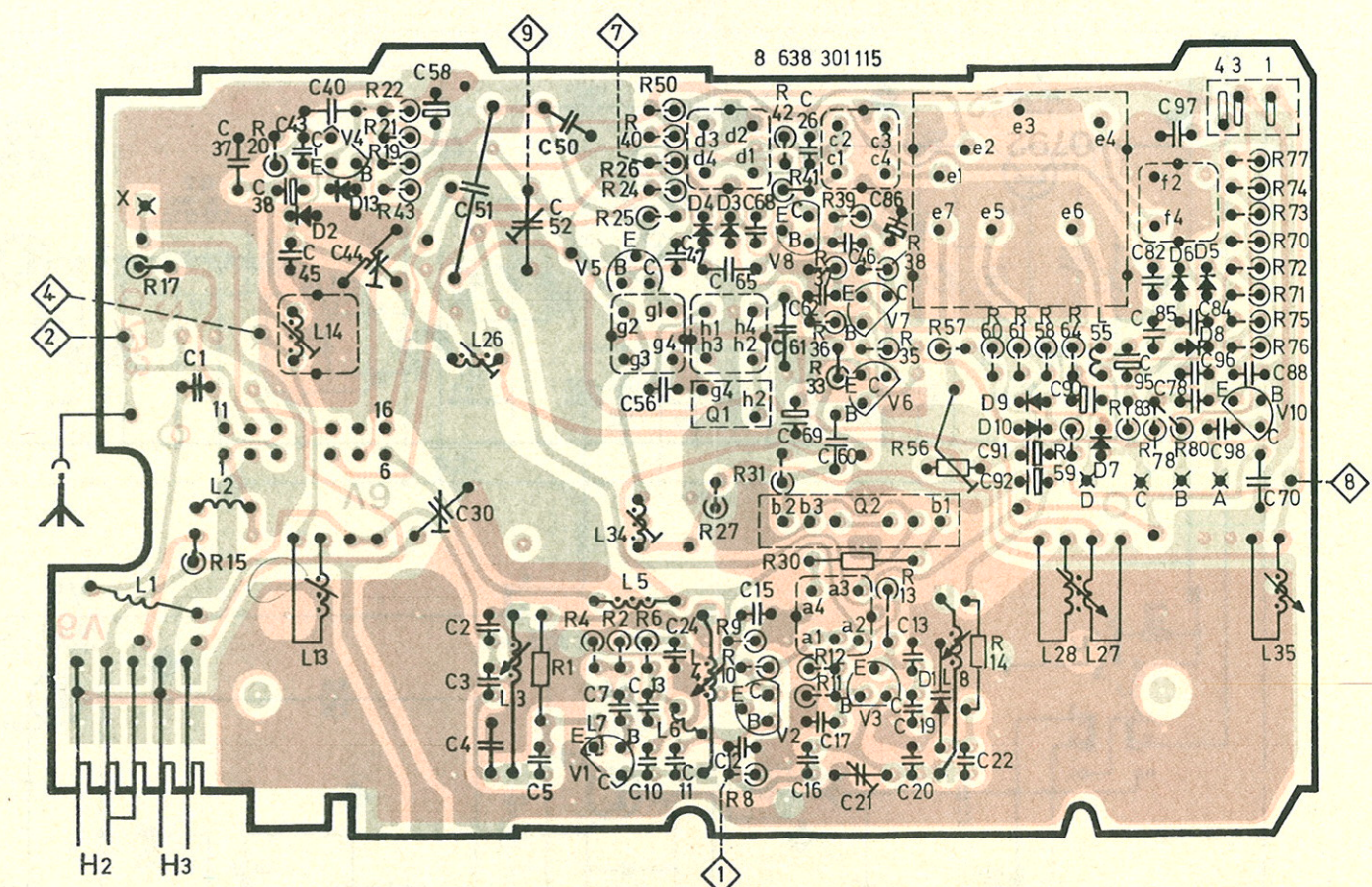
PL 1 8 638 301 115 Bedruckungsseite / Printed side / Côté imprimé / Lado impreso
