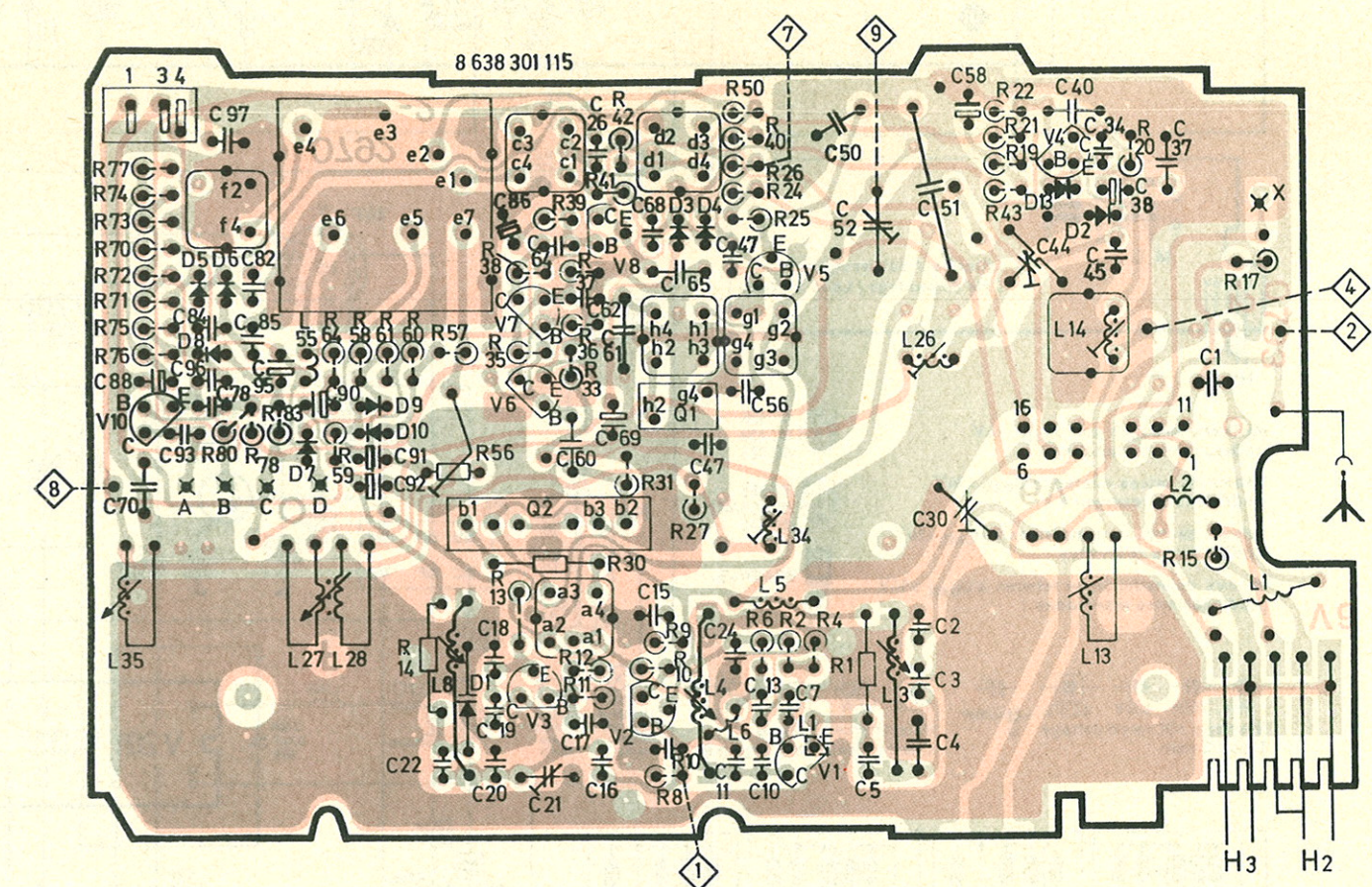
PL 1 8 638 301 115 Bestückungsseite / Components side / Côté équipement / Lado de los elementos
