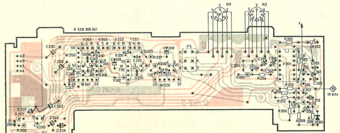
PL 2 8 638 306 041 Bestückungsseite Components side Côté équipement Lado de los elementos
